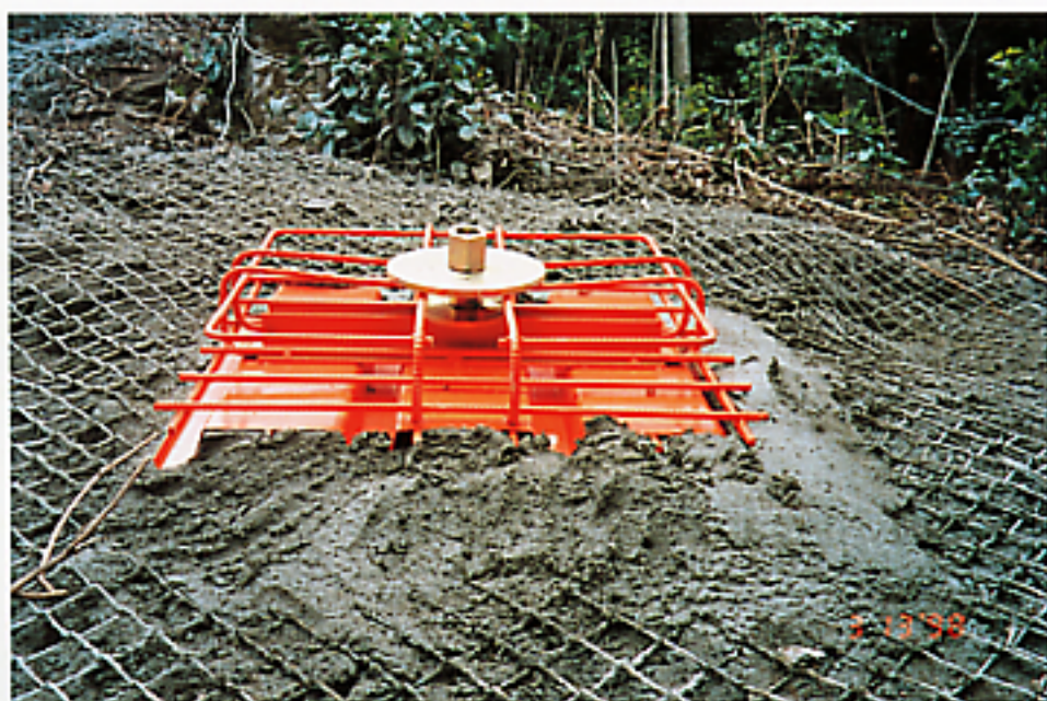
写真-1 1次支圧板実施例
